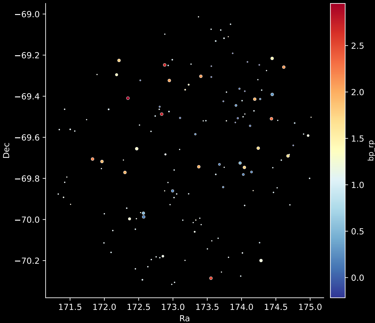
GALAH DR4 Field: [467] Stars: 149
