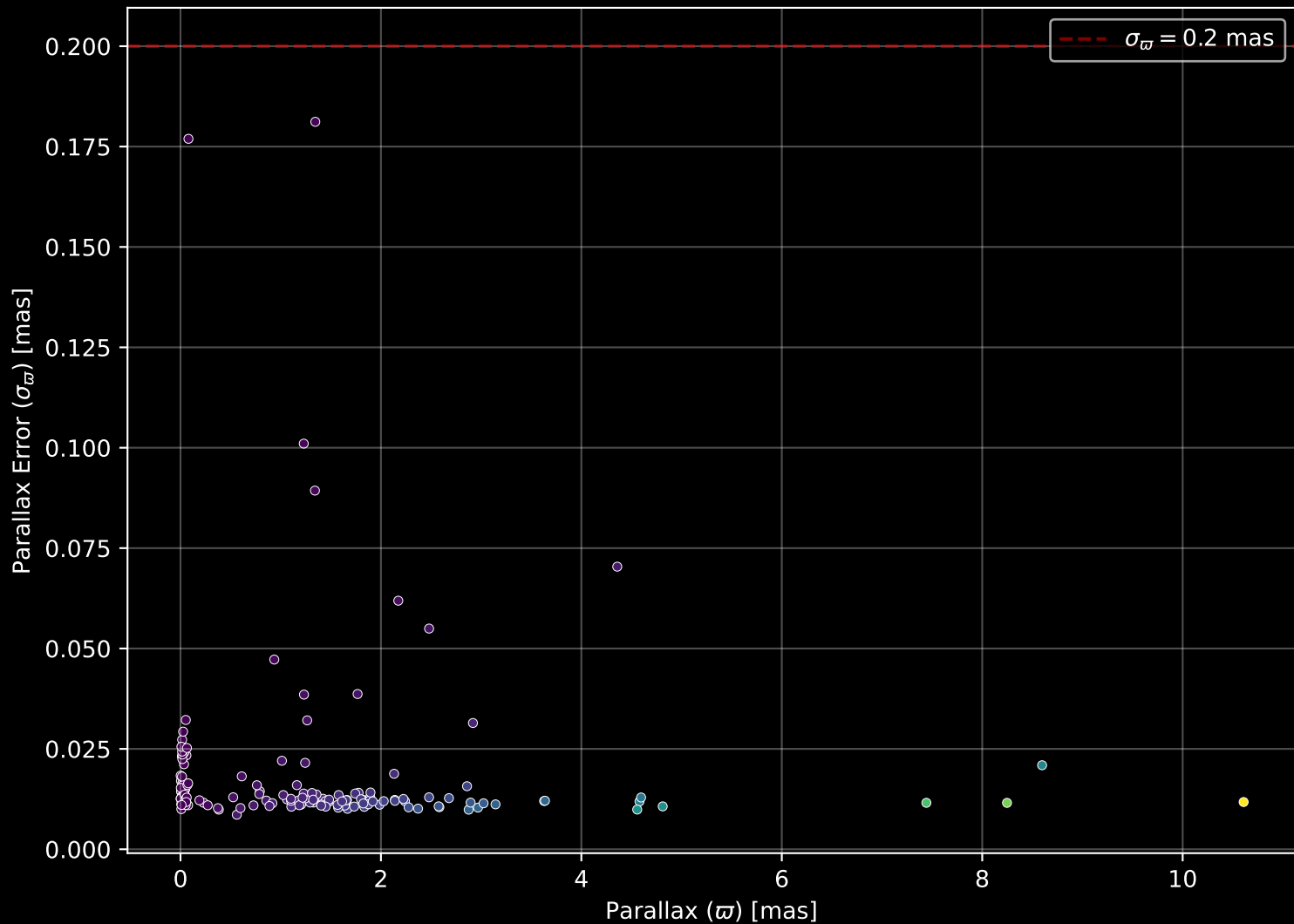
GALAH DR4 Field: [467] Parallax Quality (n= 149)
