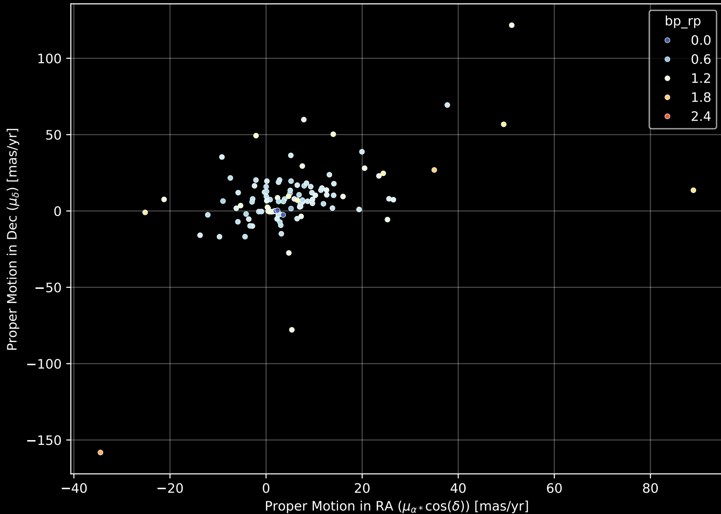
GALAH DR4 Field: [467] Proper Motion Diagram (n= 149)
