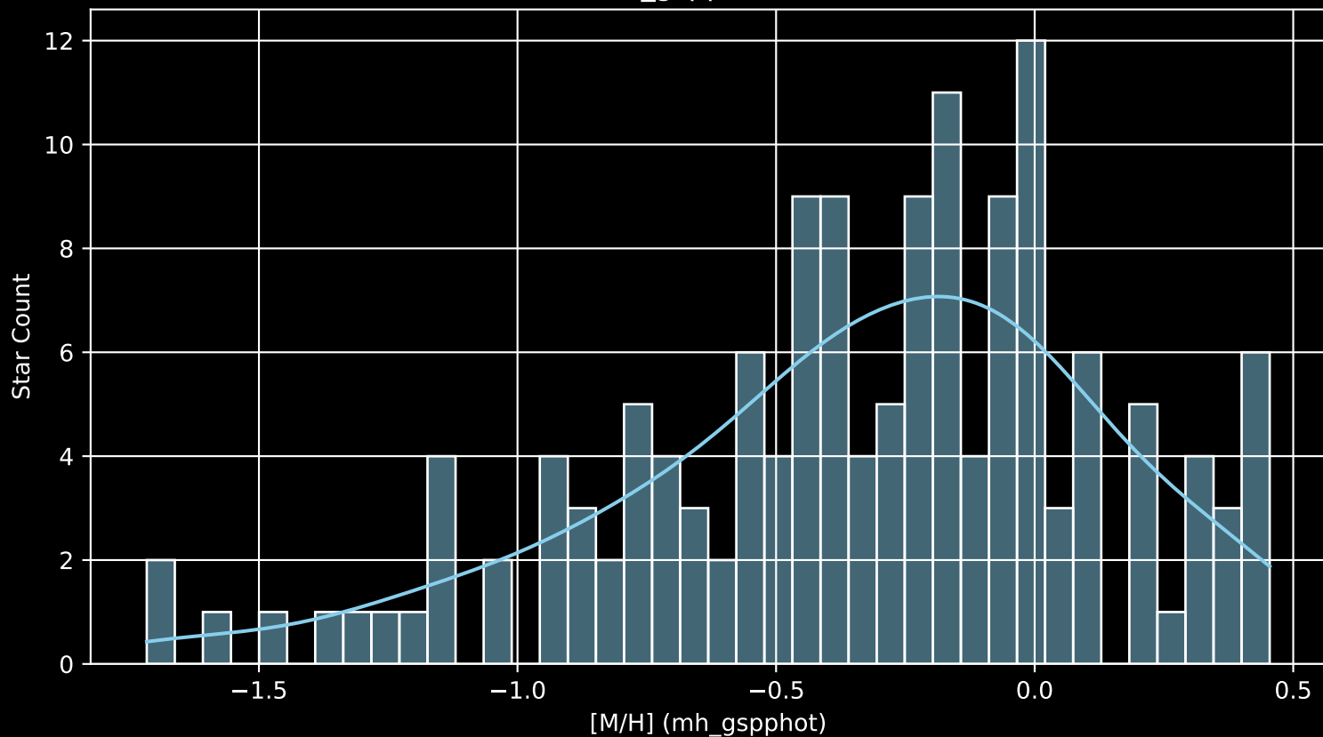
GALAH DR4 Field: [467] [M/H] (mh_gspphot) (n= 147)
