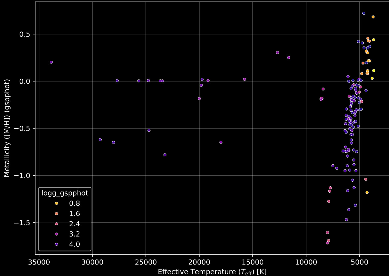
GALAH DR4 Field: [467] Stellar Population Parameters (n= 149)
